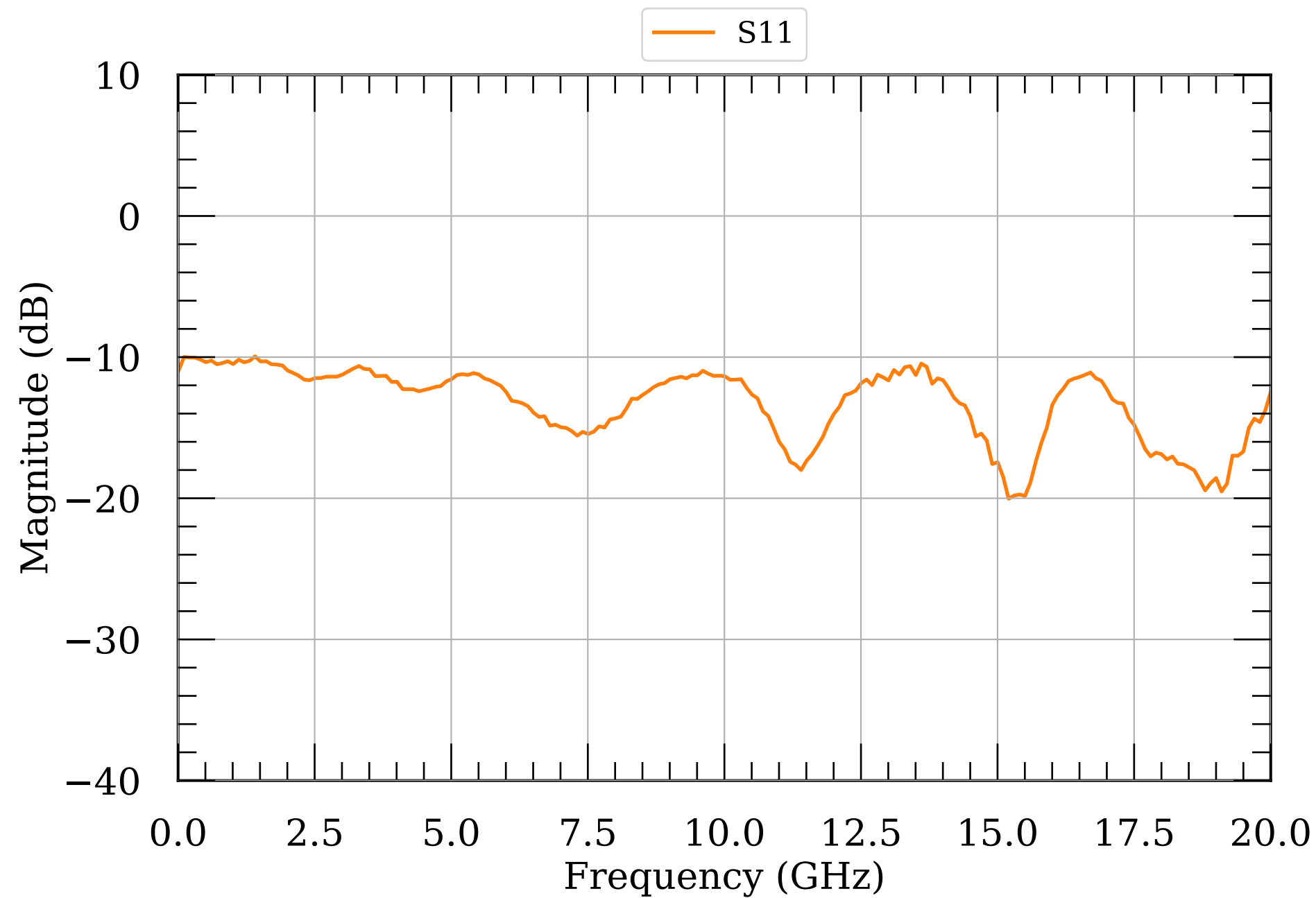
LNA S-params module074
